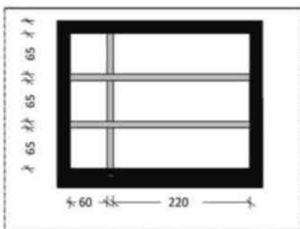
Figura 2.9 T 2 – Prerje gjatësore
