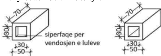
Figura 2.33 Modul i varrit mural të eshtrave
