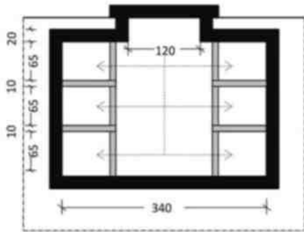
Figura 2.7 T 1 – Prerje tërthore
