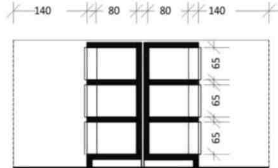
Figura 2.26 T2 –Prekje tërthore
