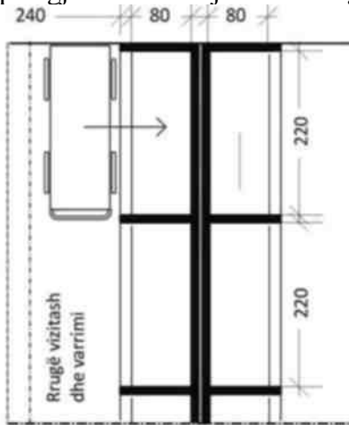
Figura 2.25 T2 – Varre murale të kufomës Planimetri
