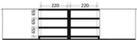
Figura 2.29 T3 – Prerje tërthore
