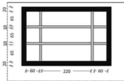
Figura 2.13 T3 –Prekje tërthore
