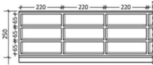
Figura 2.27 T2 – Pamje ballore
